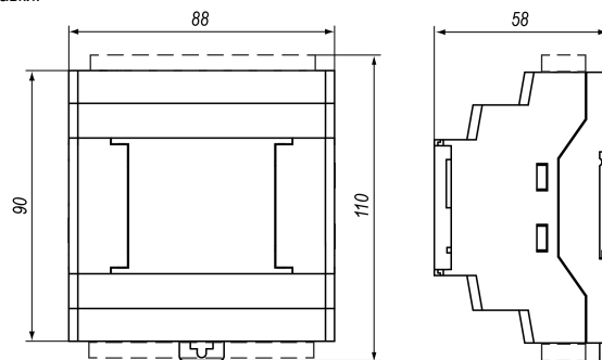
Рисунок 2 – Габаритные размеры
