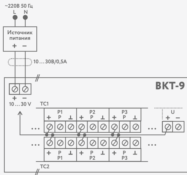
Рисунок 5.2 – Внешнее питание
