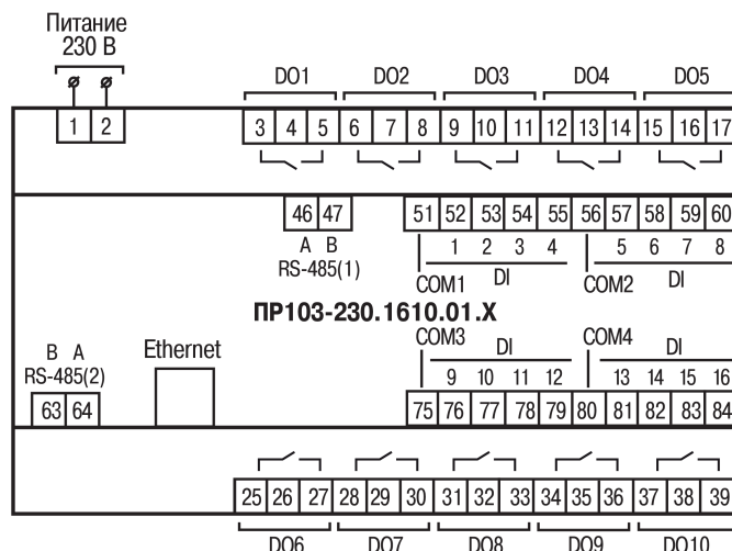
Рисунок А.1 – Расположение контактов для PR103-230.1610.01.X.0
